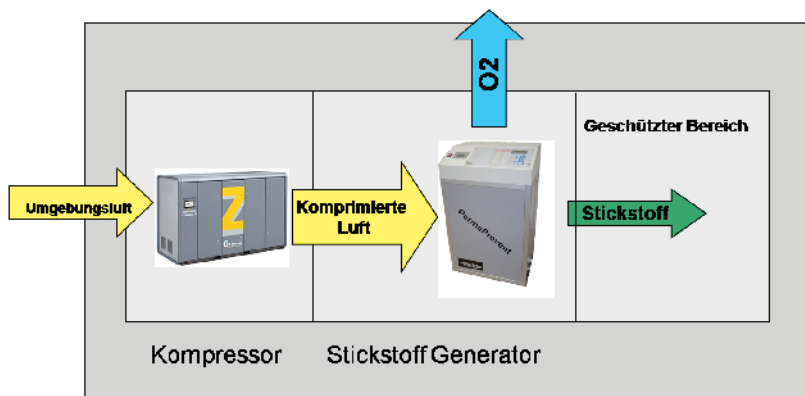
Schema eines PermaPrevent® Systems
