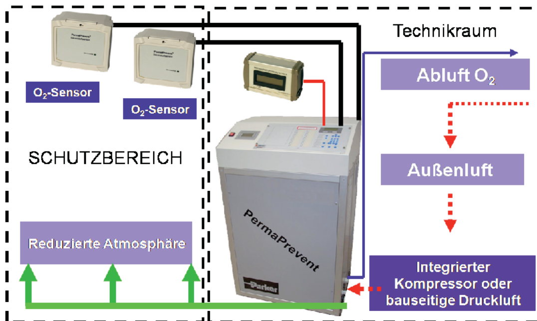
Technische Skizze
