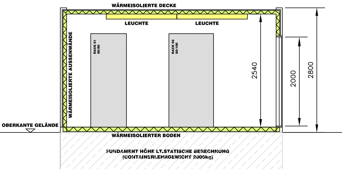
SCHNITT 1:50
