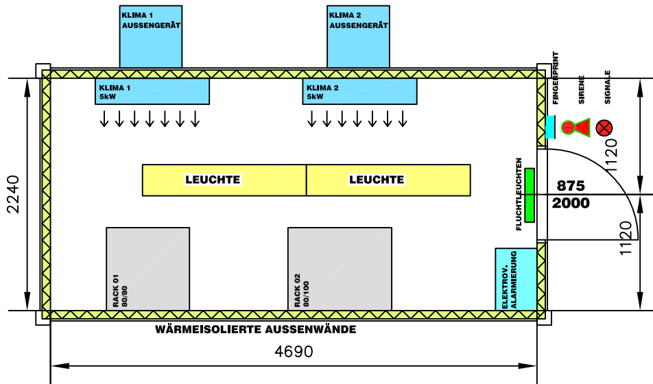
GRUNDRISS 1:50
